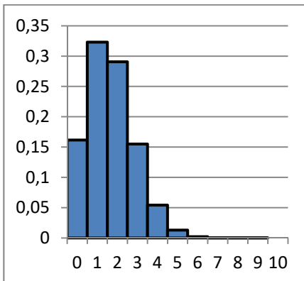
n = 10. B(10, 1/6).
