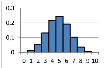
n = 10. B(10, 0.485).
