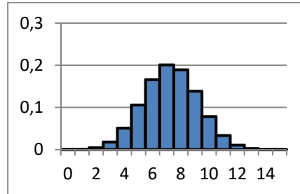
n = 15. B(15, 0.485).
