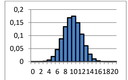
n = 20. B(20, 0.485).
