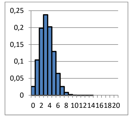
n = 20. B(20, 1/6).
