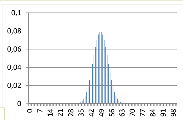
B(100, 0.485)
